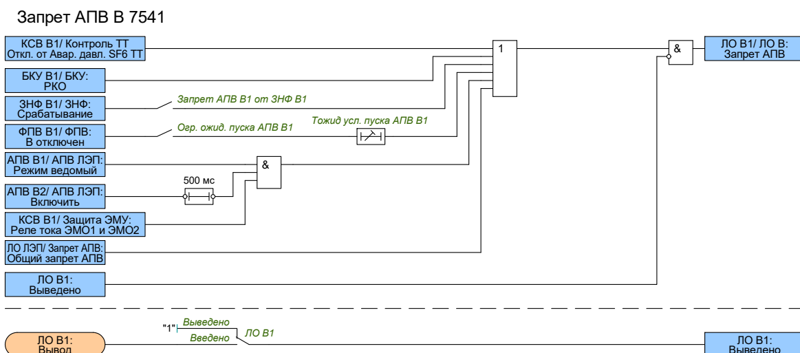
Рисунок 2.70 – Функциональная схема запрета АПВ В1
