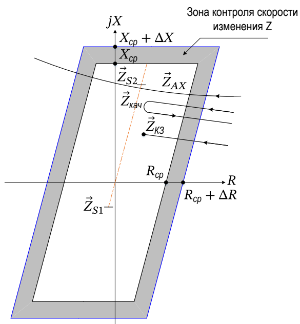
Рисунок 2.42 – Характеристики реле сопротивления, используемые для блокировки при качаниях по скорости изменения сопротивления
