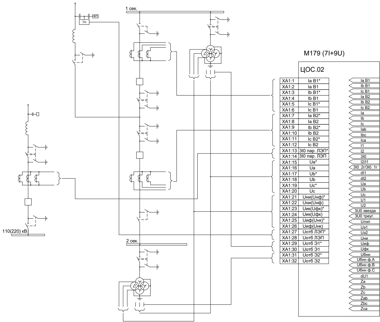
Рисунок Б.1 – Вариант подключения аналоговых цепей ТТ и ТН устройству
