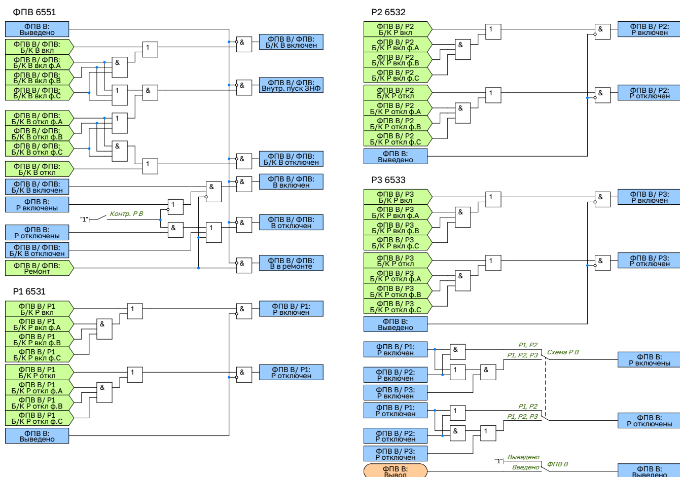
Рисунок 2.82 – Функциональная схема логики ФПВ В1
